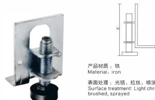
No. YGD-189 沙发脚 SOFALEGS
